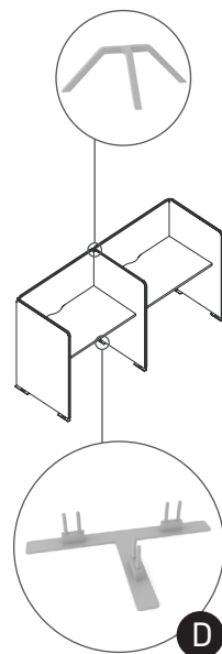
Металлическая T-образная ножка и фиксатор для передней перегородки
